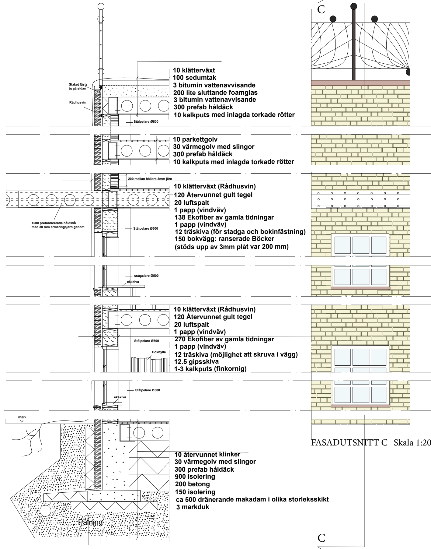
FASADSEKTION C-C Skala 1:20
